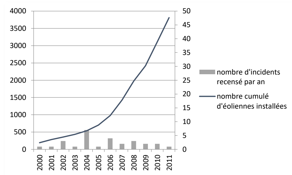
Evolution du nombre d'incidents annuels en France et nombre d'éoliennes installées
